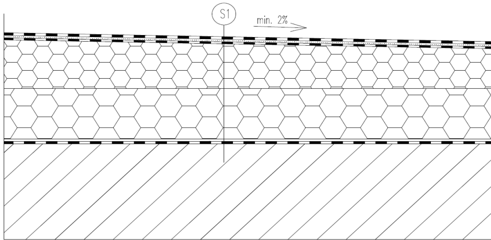
Řez střešní konstrukcí
