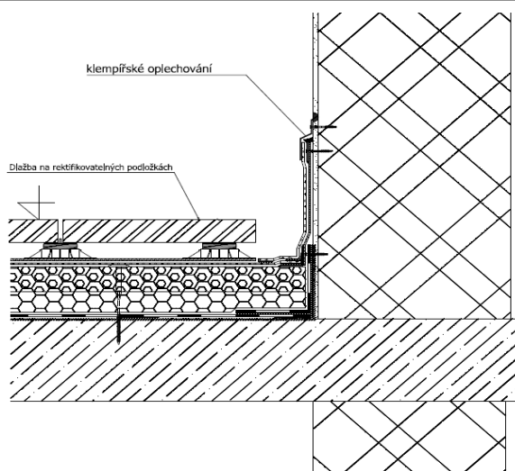
Detail ukončení hydroizolace u stěny
